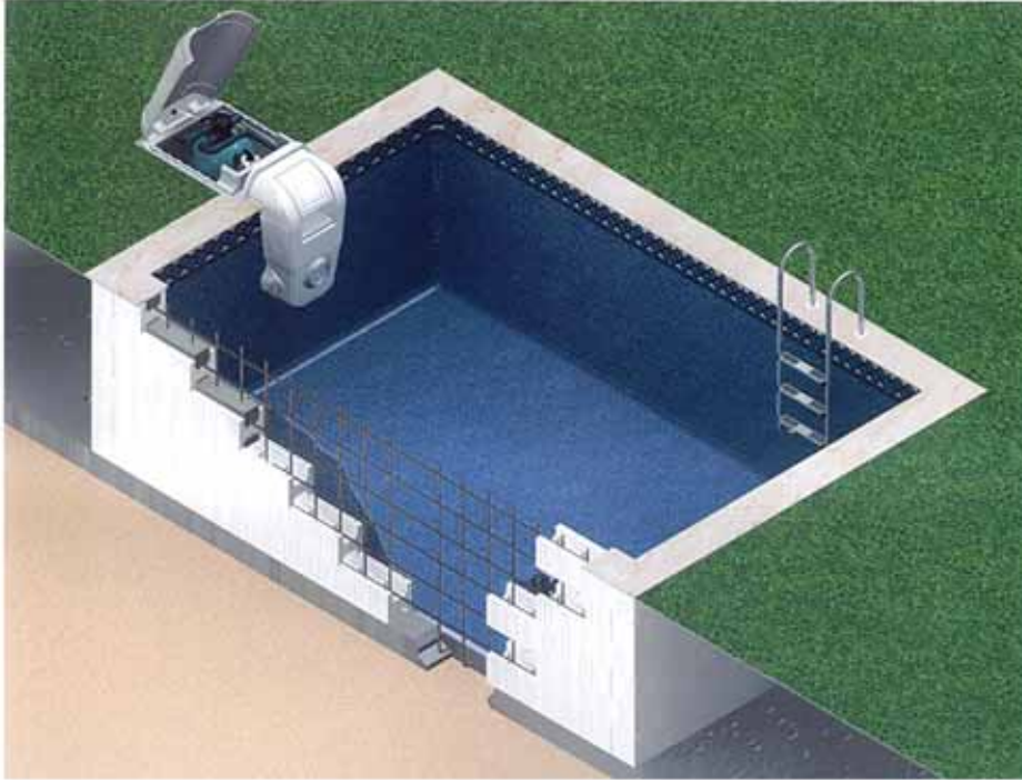
Stropool RECTON-LD ( iniş merdiveni, 17401, opsiyoneldir. )
