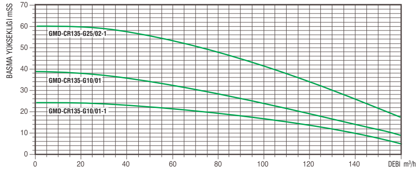
PERFORMANS EĞRİLERİ
