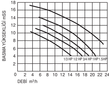
PERFORMANS EĞRİLERİ
