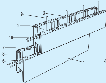
Şekil 1: İki adet stropor bloğun üst üste dizilmesi
