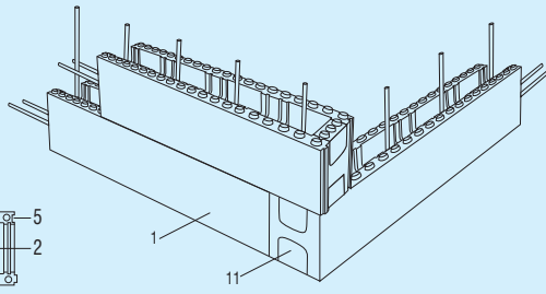
Şekil 3: Stropor bloğun köşe dönüşlerde dönüş birleşimi
