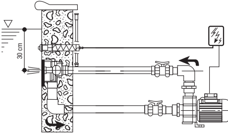
MONTAJ ŞEMASI:
