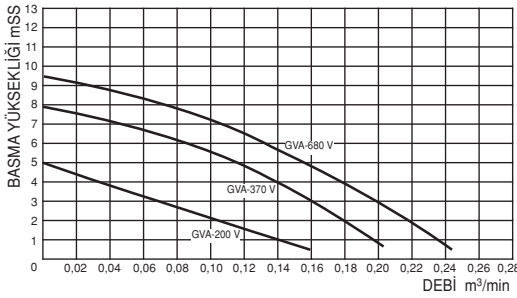
PERFORMANS EĞRİLERİ
