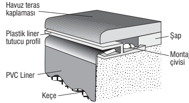
Liner askı profiline bağlantı şekli
