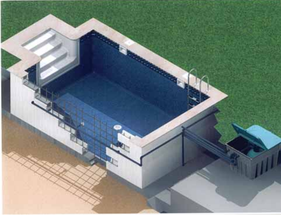
Stropool RECTON-SL ( iniş merdiveni, 17401, opsiyoneldir. )
