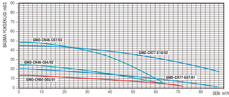
PERFORMANS EĞRİLERİ
